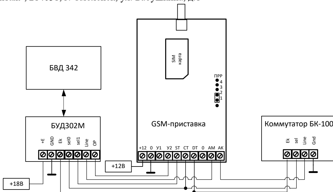
Подключение приставки в схеме с коммутатором
