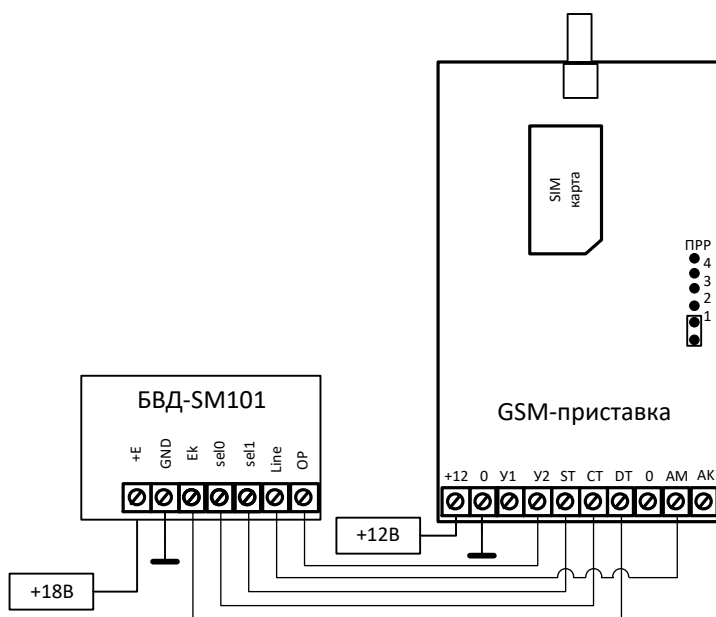
Подключение приставки в схеме без коммутатора
